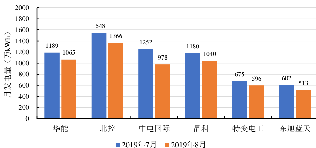
图3 新泰基地各项目月发电量
