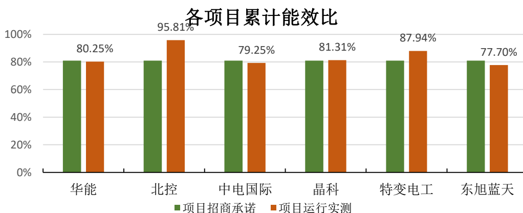
图 9 新泰基地各项目当年累计能效比对比
