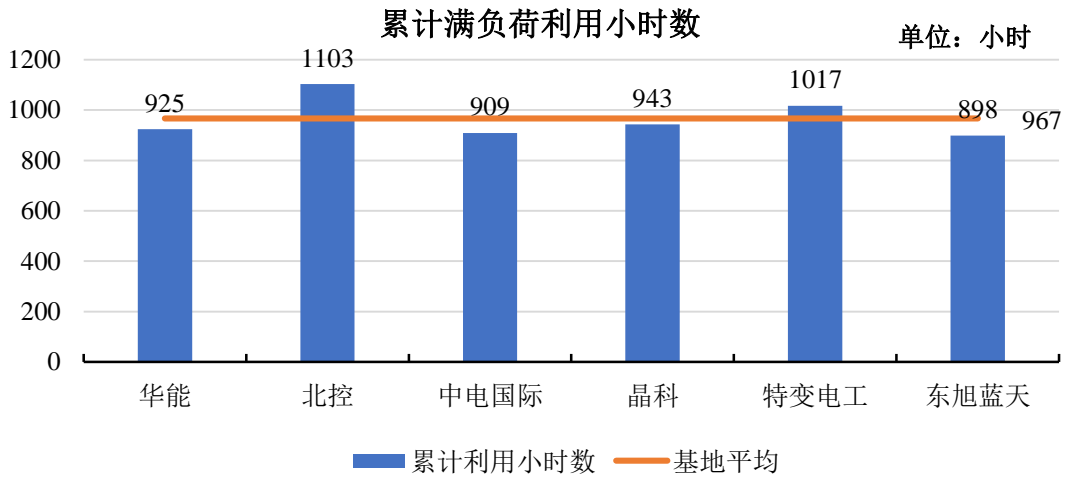
图 5 新泰基地各项目累计满负荷利用小时数
