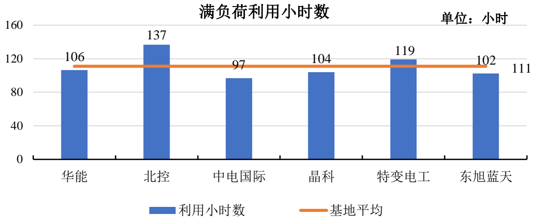
图 4 新泰基地各项目月满负荷利用小时数
