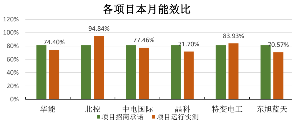
图 8 新泰基地各项目能效比对比
