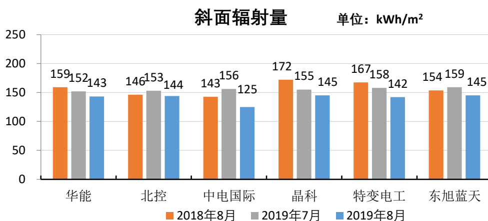
图 2 新泰基地各项目月斜面辐射量
