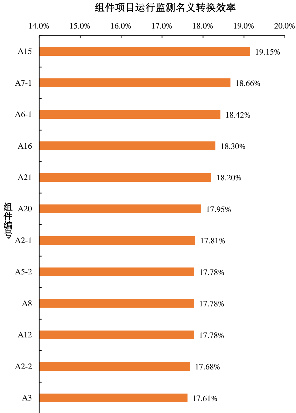
图 6 新泰基地组件项目运行监测名义转换效率
